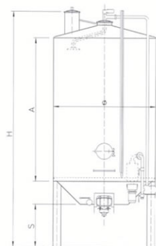
■ Schema del vinificatore VSE.
